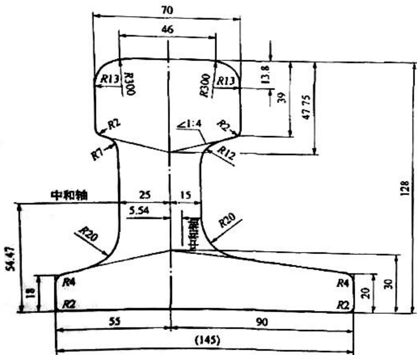
图 1 50 AT 钢轨断面
